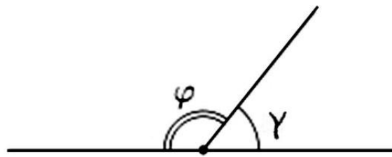
Смежные углы
