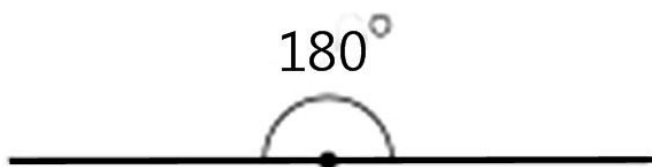
Развёрнутый угол
